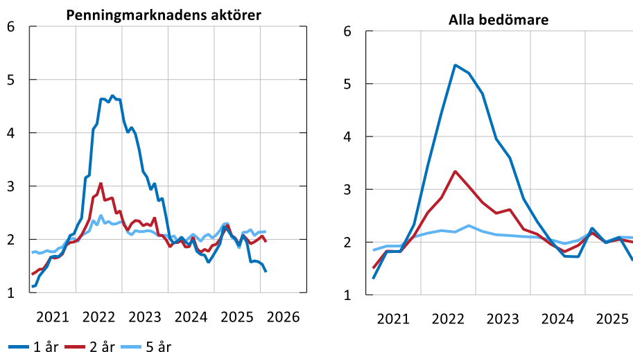
Diagram 35. Inflationsförväntningar Procent
